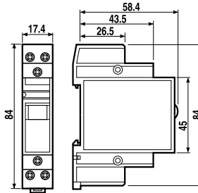
Тип 22.24 Винтовой клеммы
