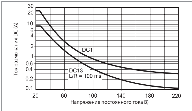
Н 66 - Макс. отключающая способность DC
