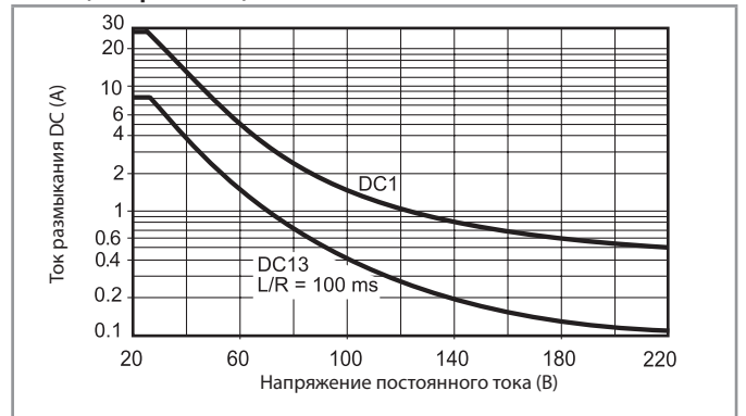
Н 66 - Макс. отключающая способность DC, х60х версии (зазор >1.5 мм)
