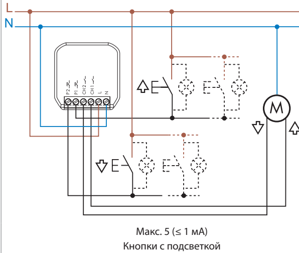
Тип 13.S2 4-проводное соединение
