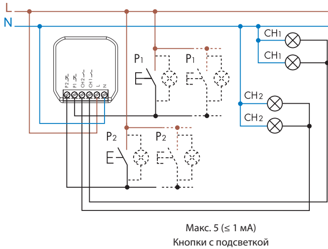
Тип 13.72 4-проводная схема
