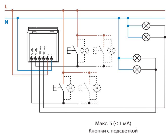
Тип 13.72 4-проводная схема
