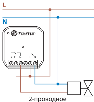
Тип 13.21.8.230.S000 Подключение соленоида по 2, 3 и 4 проводам или прямое подключение
